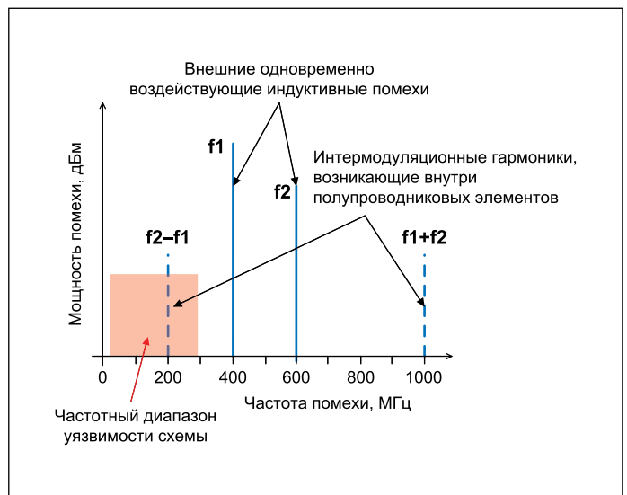
Рис. 2. Возникновение интермодуляционных гармоник в «уязвимом» частотном диапазоне системы
