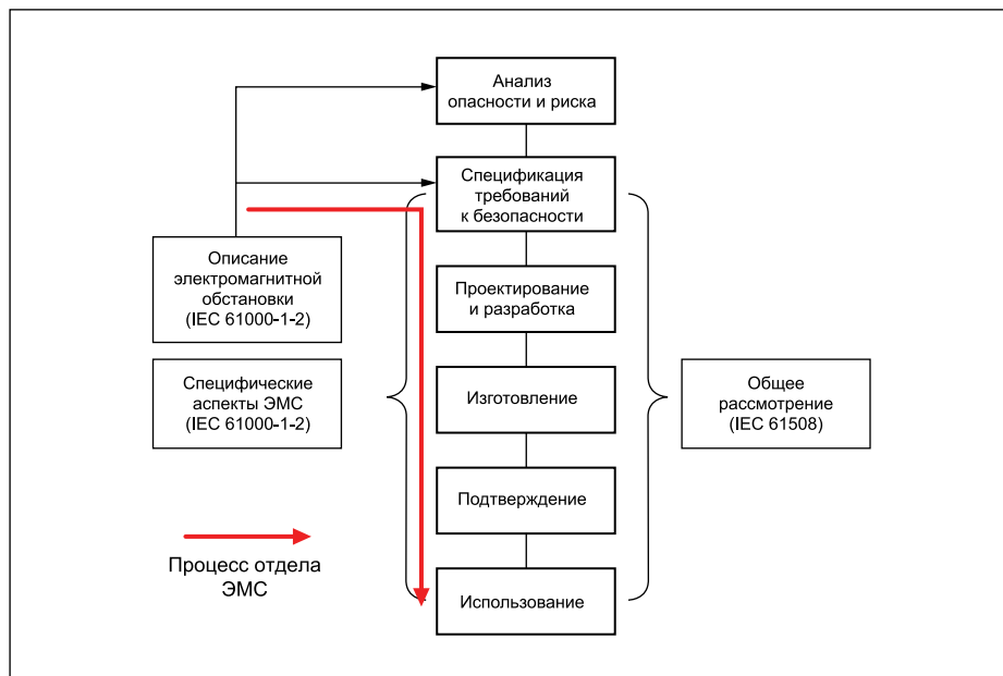
Рис. 6. Процесс обеспечения безопасности в отношении электромагнитной совместимости в соответствии с ГОСТ IEC/TS 61000-1-2-201
