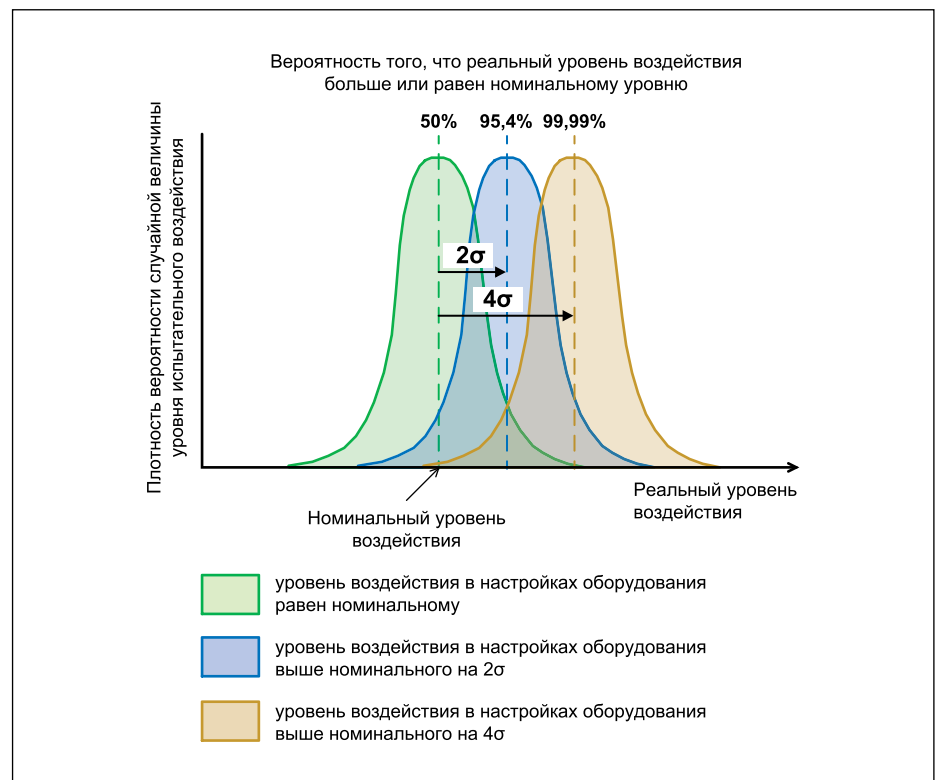
Рис. 5. Повышение номинального уровня испытательного воздействия для увеличения доверительной вероятности результатов испытаний
